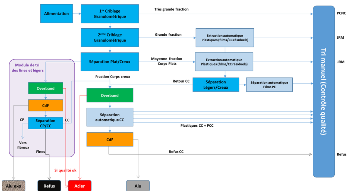
Figure : Synoptique fonctionnel d'un process de tri
