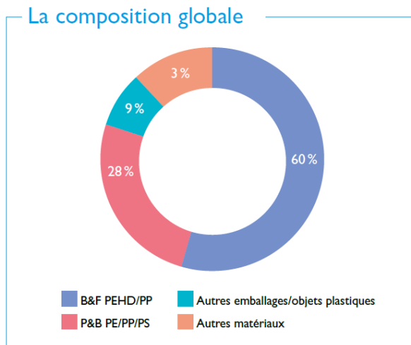
PEHD-PP-PS
